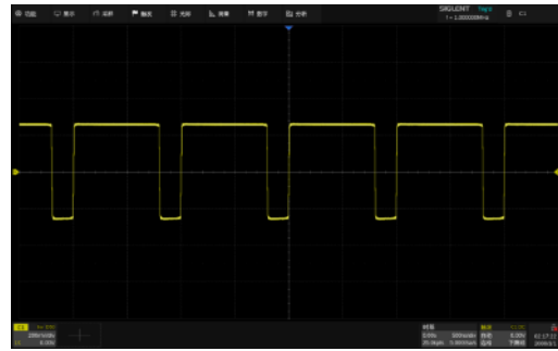
反相开启
