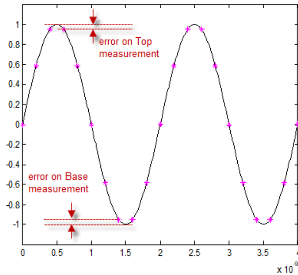
采样不足引起的垂直测量误差
