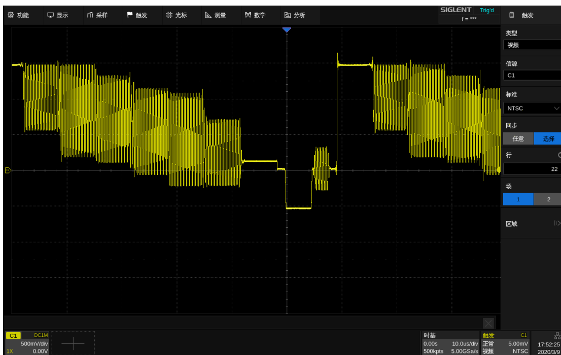
特定行上视频触发（NTSC 标准）
