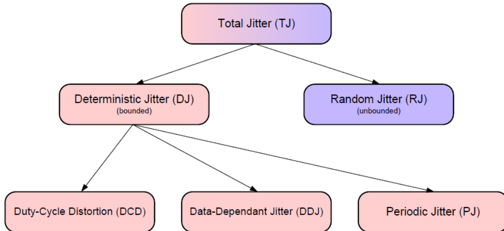
图 31.1 抖动的分解
